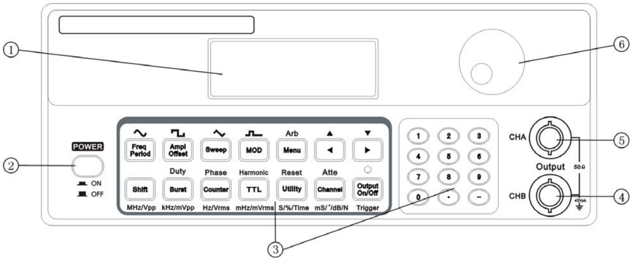
前面板
