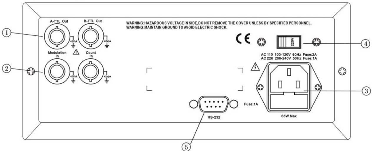
後面板
