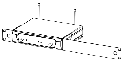
安裝 1 台接收機
