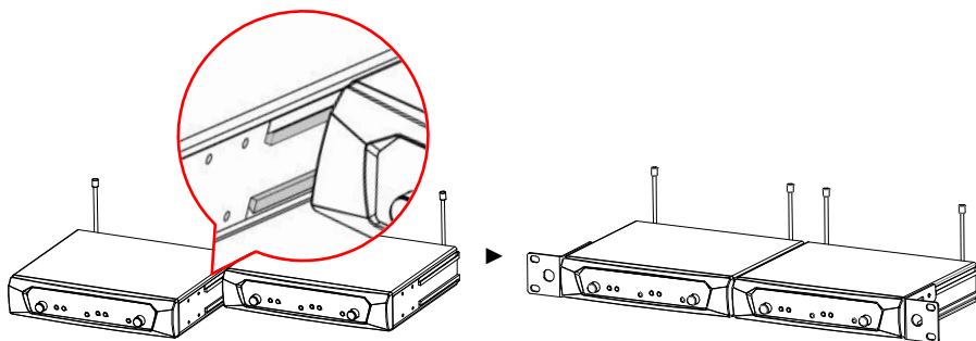
安裝 2 台接收機
